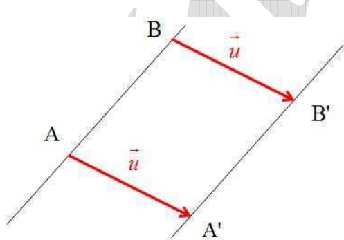
Translation de vecteur \vec{u}
