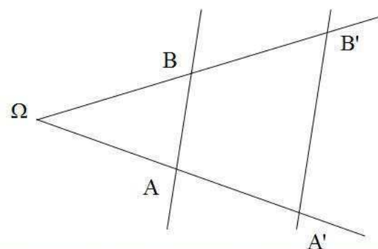
Homothétie de centre \Omega et de rapport k > 0 .
